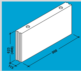
KS-PE 115
