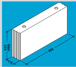
KS-PE 175
