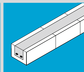
KS - Hinter- und Sichtmauerstürze
